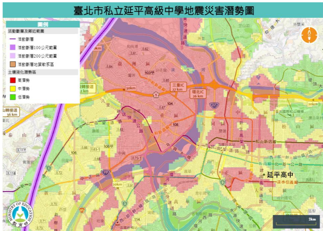
圖 2.4.1 地震災害潛勢圖 (瀏覽日期：113 年 9 月 6 日)
